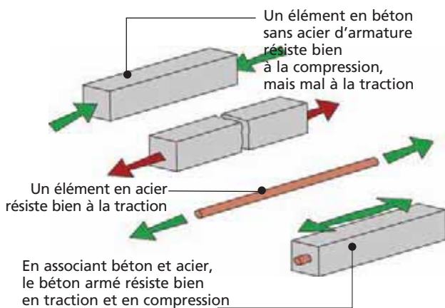
Principe du béton armé
